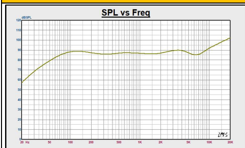
频响曲线
