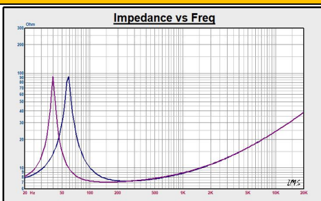
阻抗曲线
