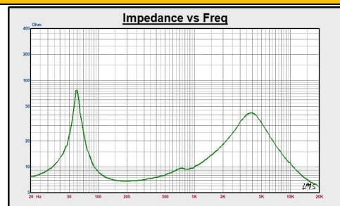
阻抗曲线
